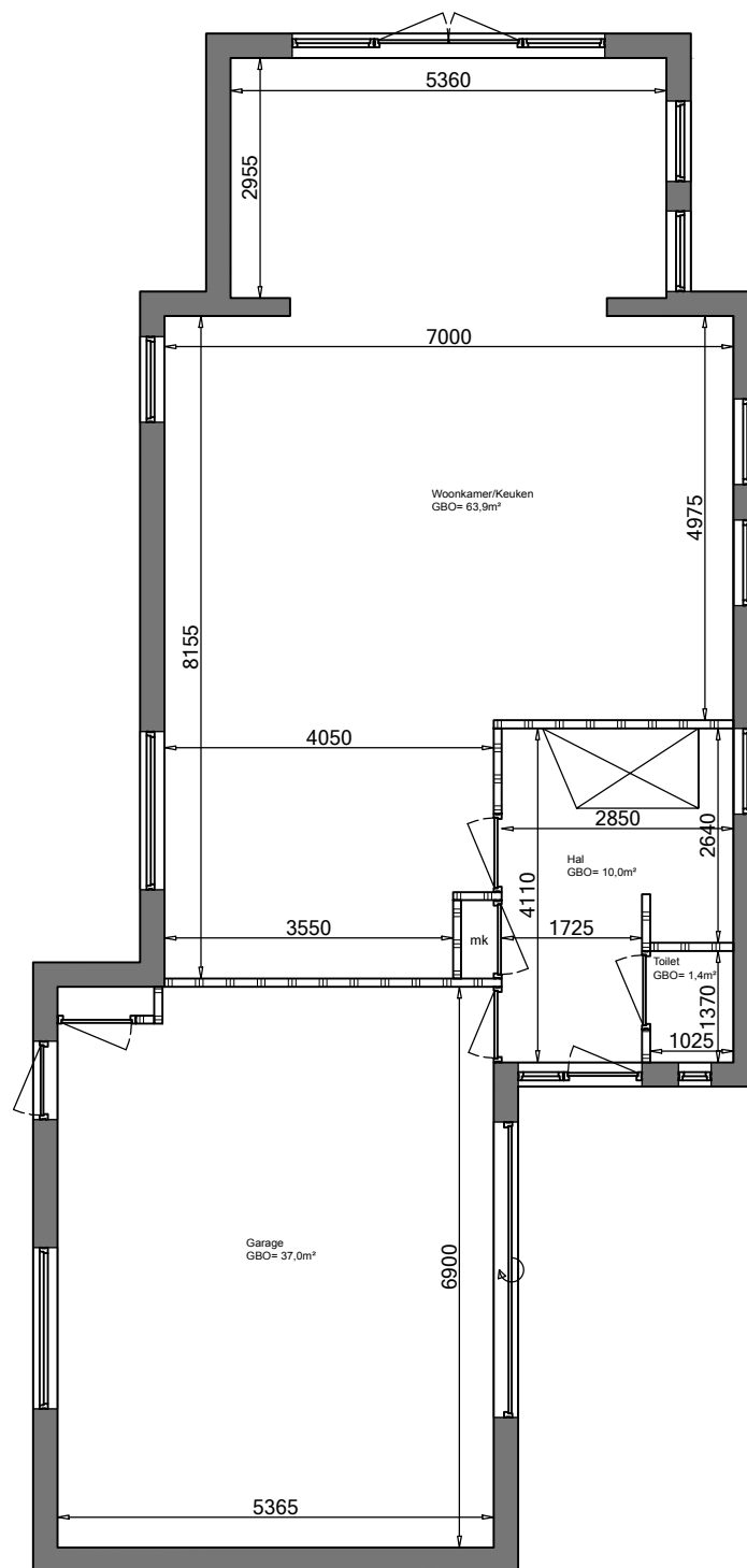
Begane grond
